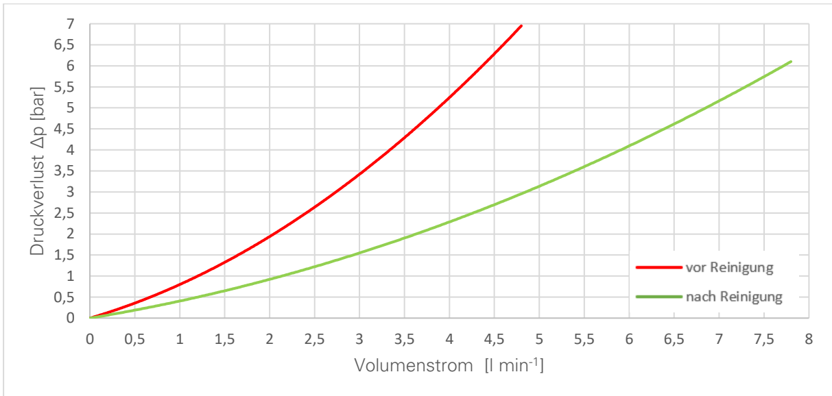
Abbildung 6: Anlagenkennlinie eines Werkzeug-Kühlkanals
