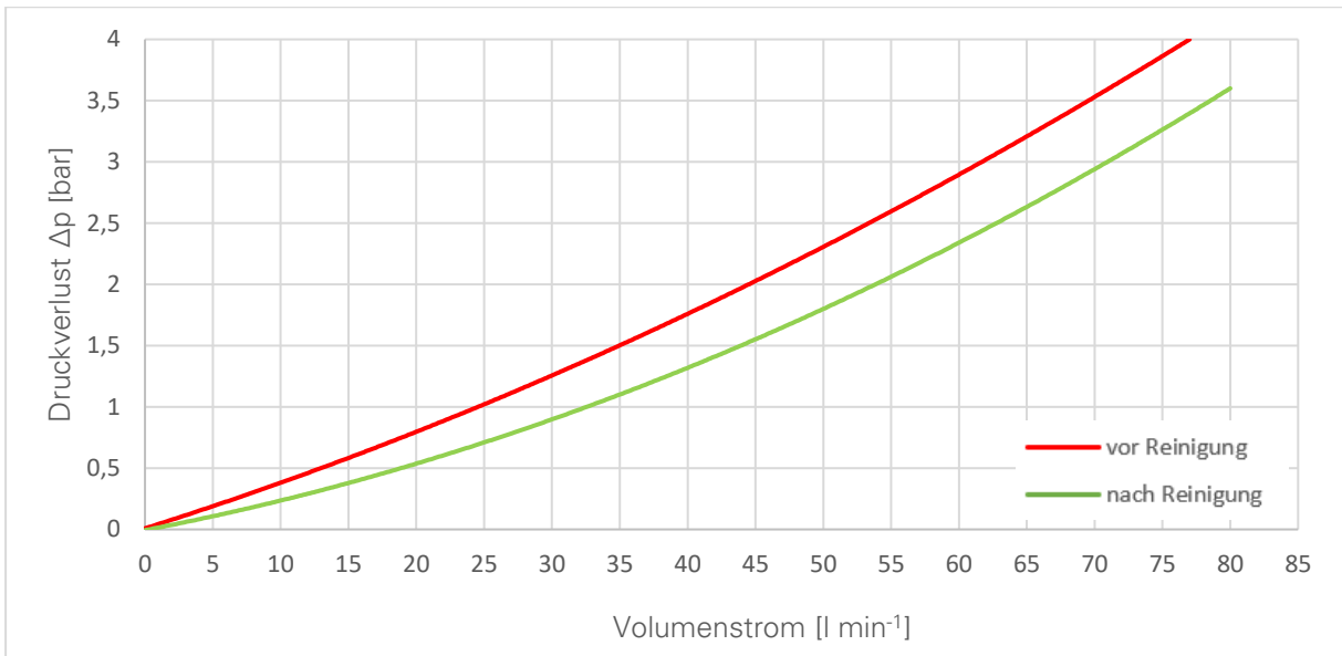
Abbildung 5: Systemkennlinie einer Werkzeugseite
